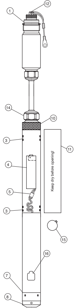
DCX-22SG-CTD
