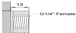
G 1/4" Female DIN EN ISO 228
