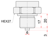
G1/2" B EN 837-1
